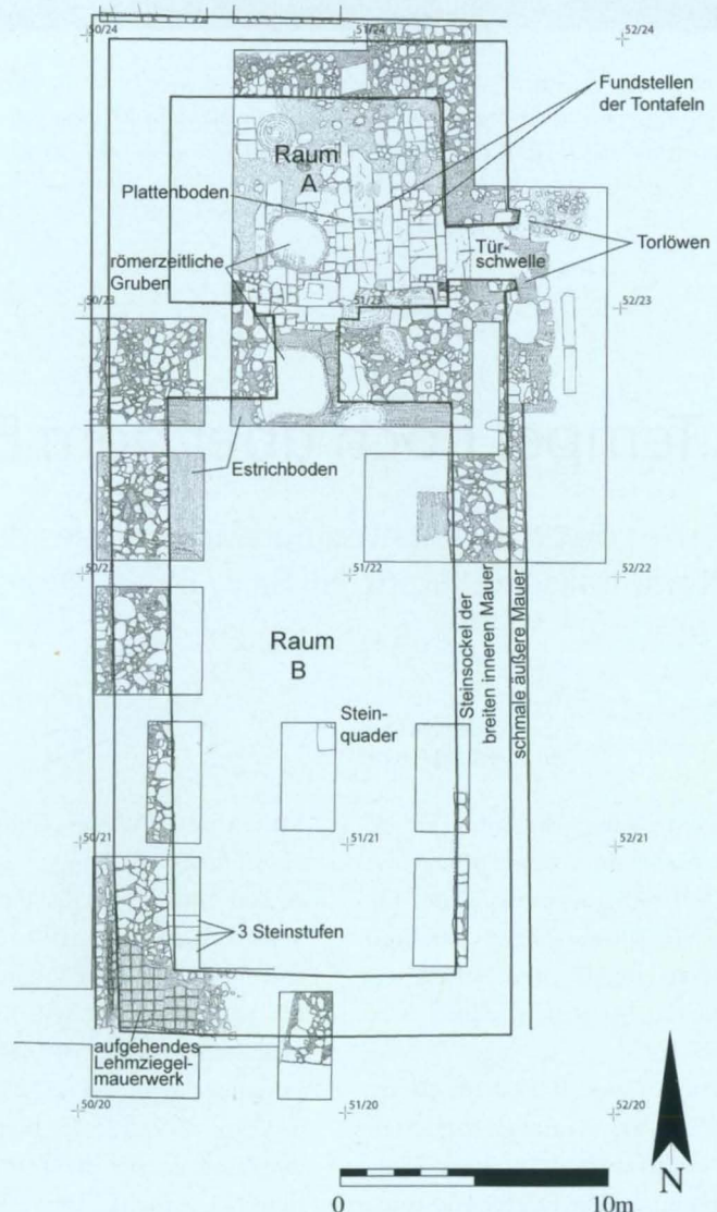
Abb. 3 Grundriß des Tempels auf der Zitadelle von Bazi. Der kleinere Raum A im Norden ist im Gegensatz zu dem größeren Raum B mit mächtigen Steinplatten gepflastert. Mit 38 m Länge und 16 m Breite gehört der Bau zu den größten Tempeln des bronzezeitlichen Syrien.
