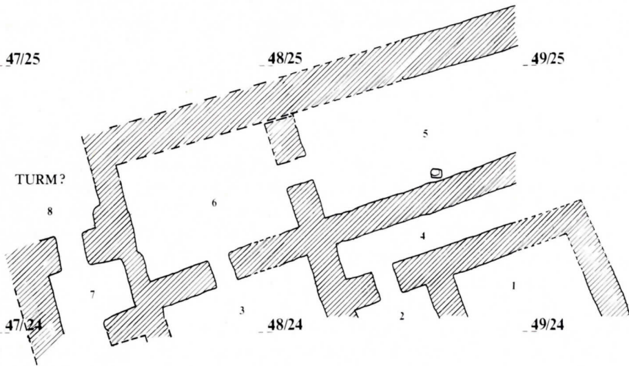
Abb. 7: Zitadelle, römische Befestigung, schematische Übersicht (Maßstab 1 : 200)
